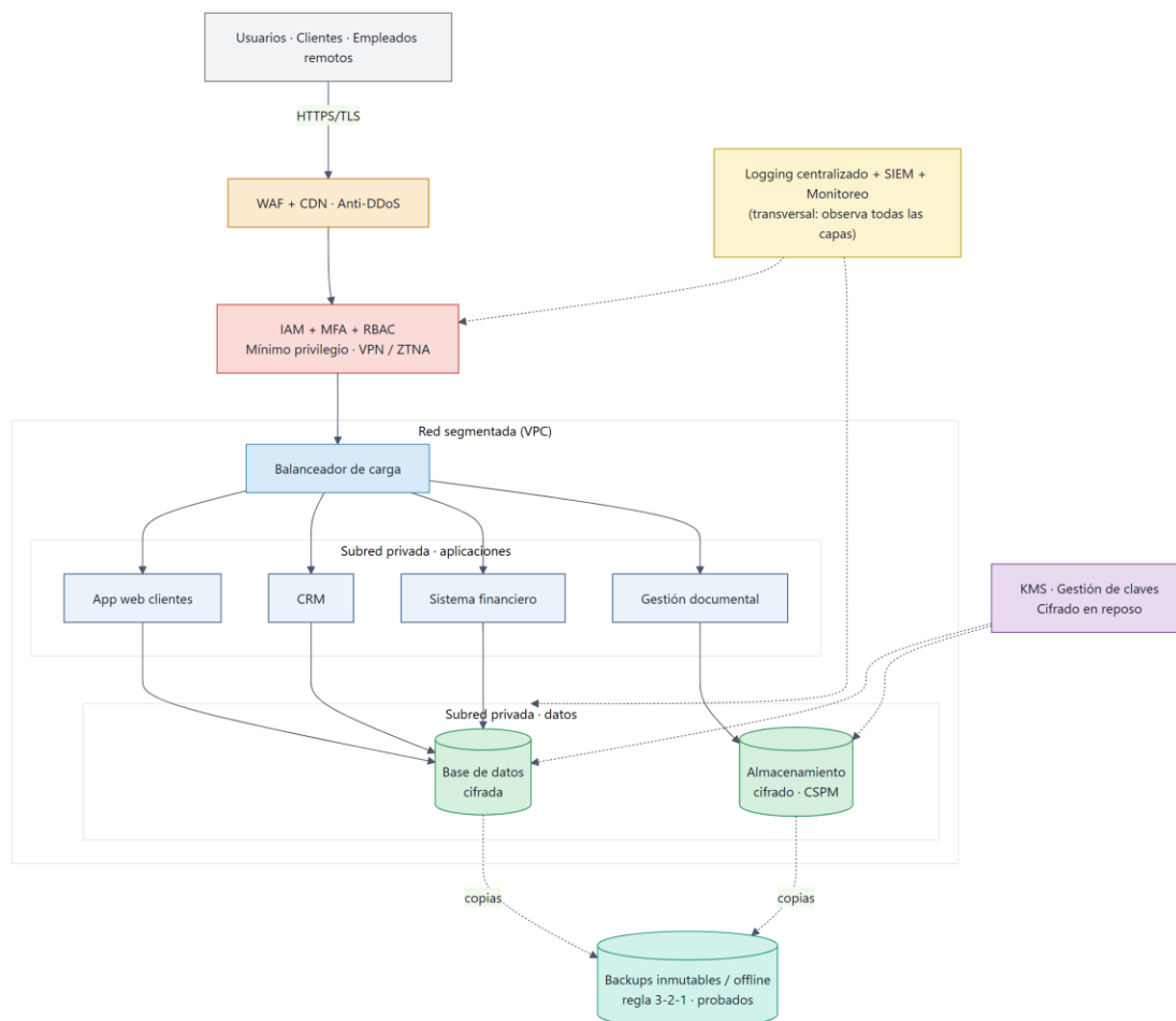
Figura 2. Arquitectura de seguridad cloud propuesta: el tráfico entra por un WAF/CDN, se autentica con IAM + MFA, atraviesa una red segmentada (VPC) con subredes separadas para aplicaciones y datos, con cifrado gestionado por KMS, copias inmutables fuera de línea y monitoreo (SIEM) transversal.
